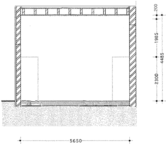
Dwarsdoorsnede / cross section naar achteren gezien / towards the back
