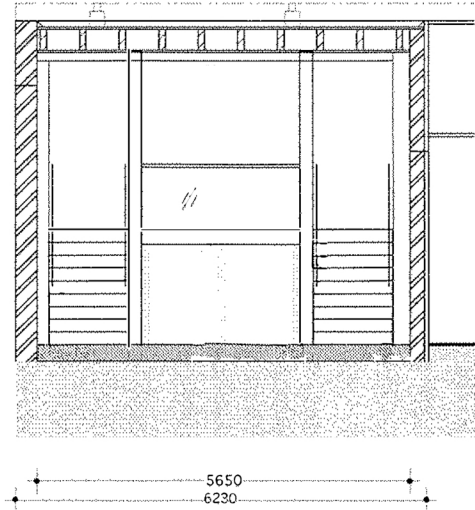
Dwarsdoorsnede / cross section naar voren gezien / towards the front
