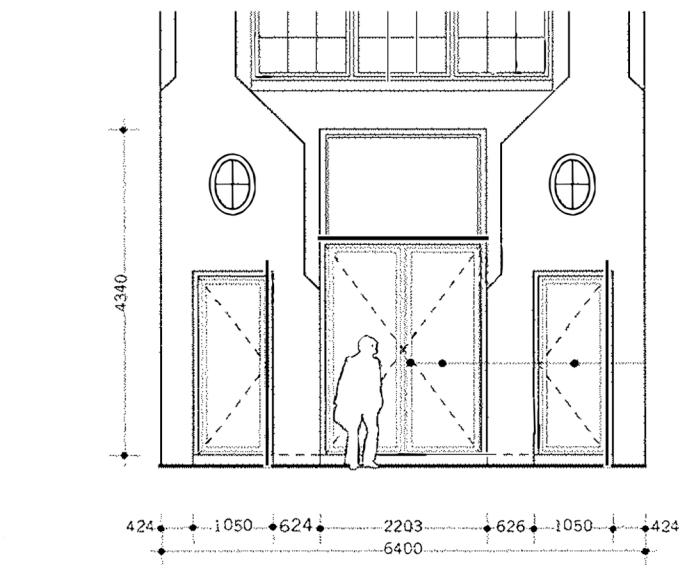
Aanzicht voorgevel / front facade view
